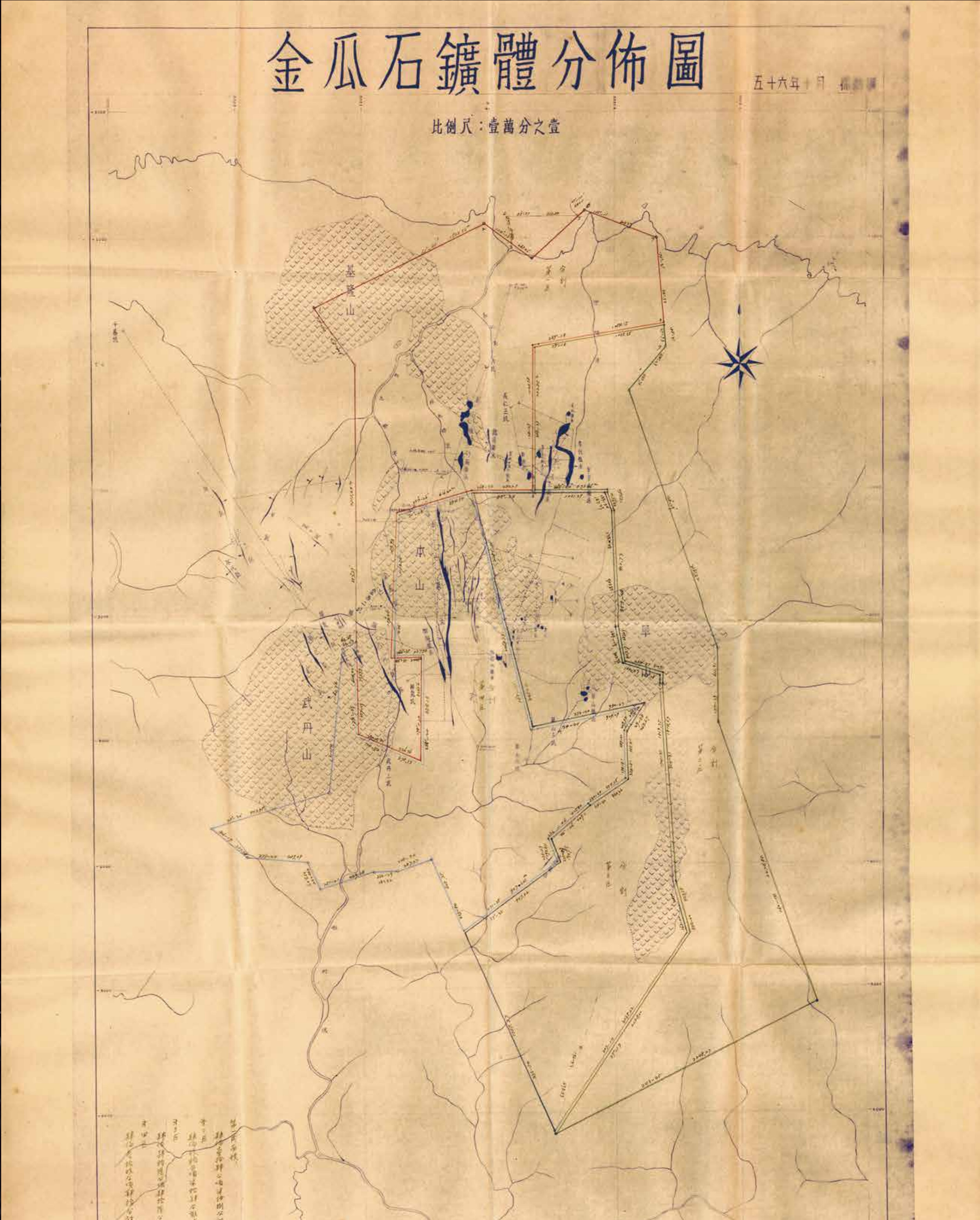
↑ 1967 年金瓜石鑛體分布圖 分區標示各礦床在金瓜石本山、武丹山的位置。 1967 A313380000K/0056/205/007 國家發展委員會檔案管理局
