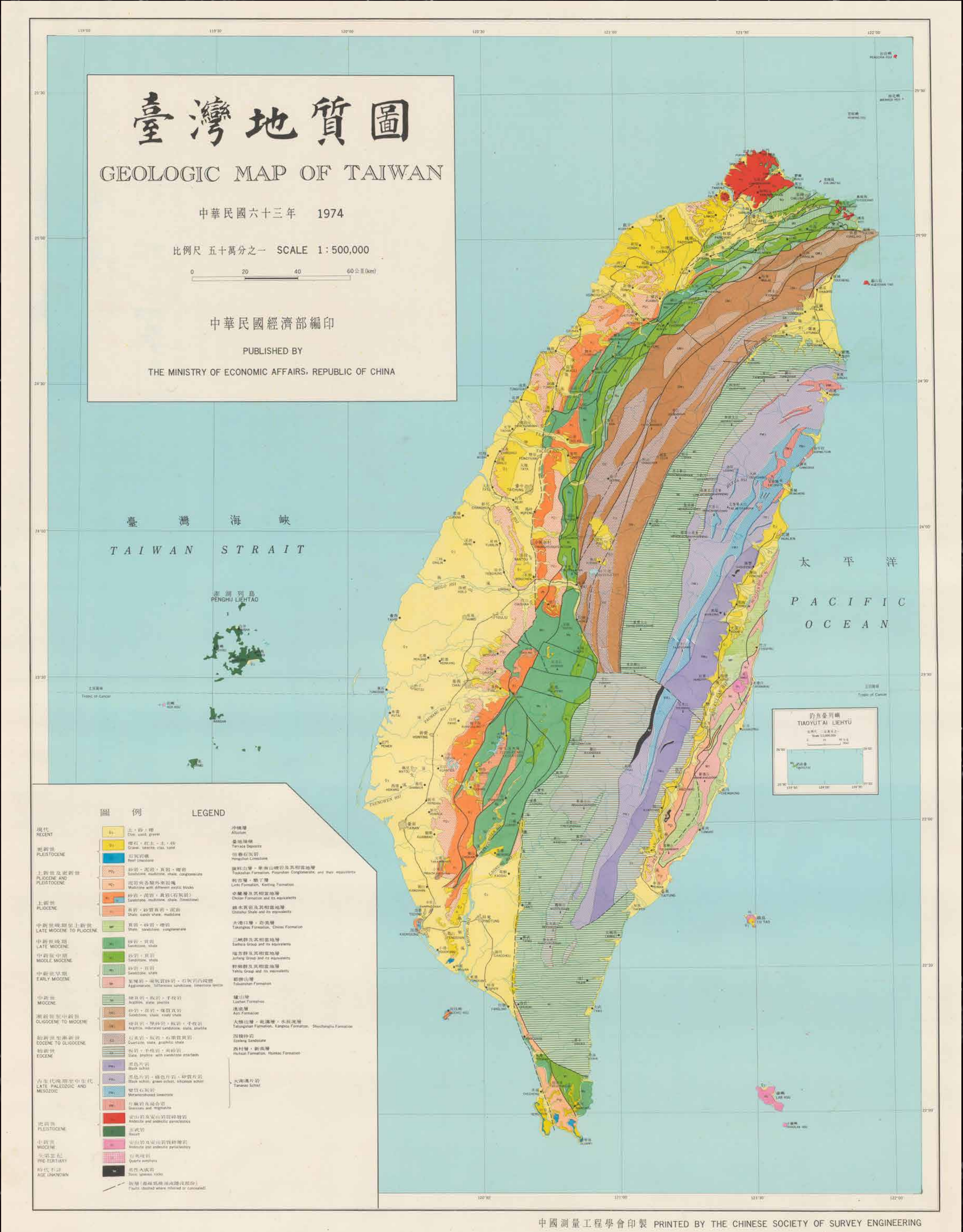
↑ 1974 年臺灣地質圖 基隆山、本山、九份等地的安山岩區主要為石英安山岩，蘊藏之主要礦物為自然金、硫砷銅礦與黃鐵礦等。 1974 A313380000K/0063/205/001 國家發展委員會檔案管理局
