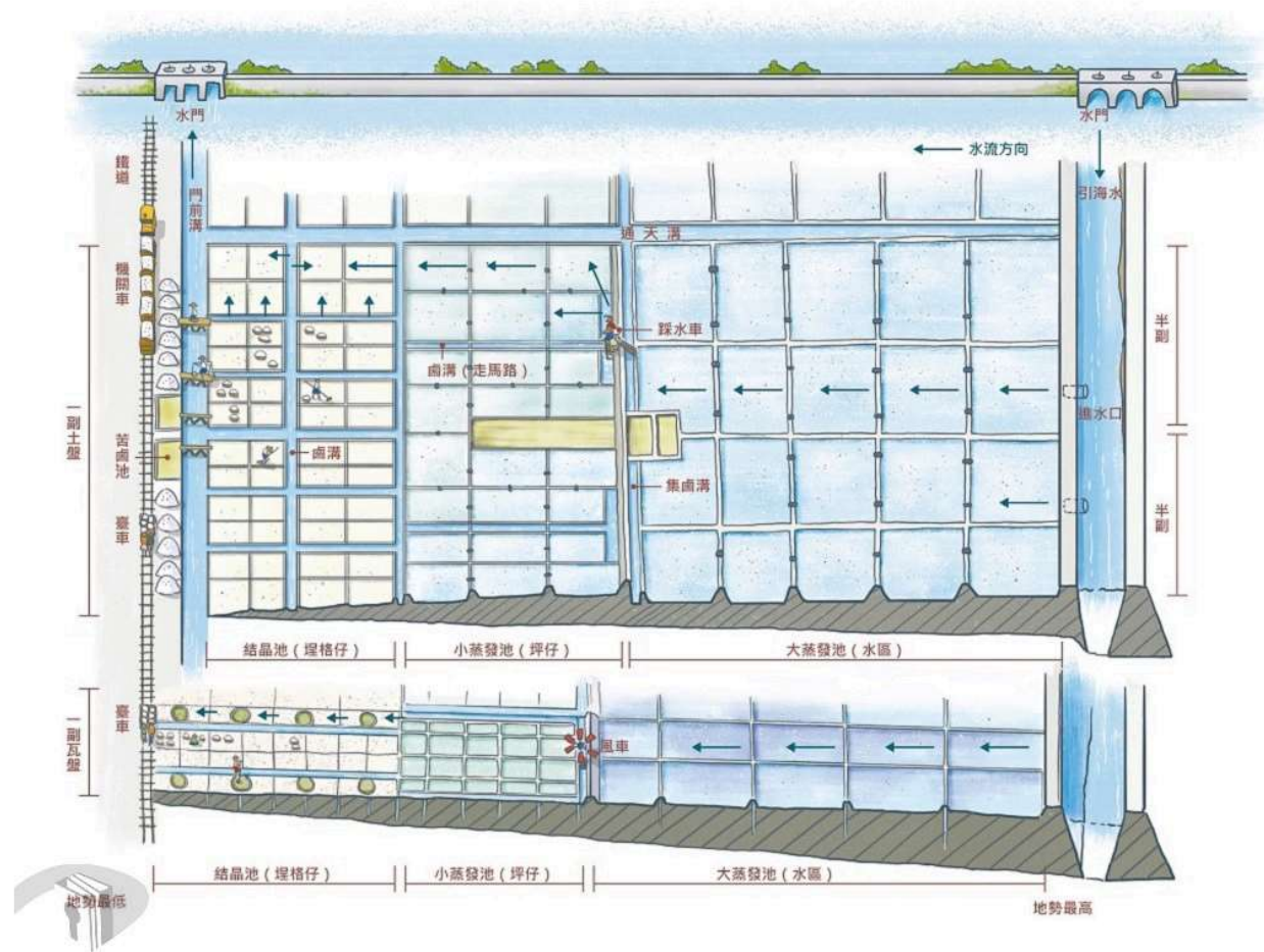
圖2 曬鹽流程图
