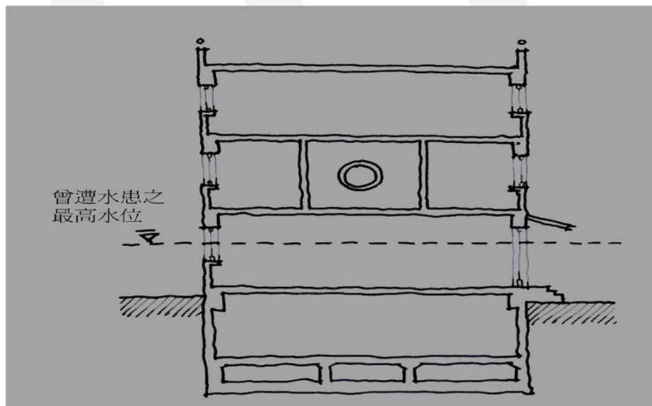
剖面圖
