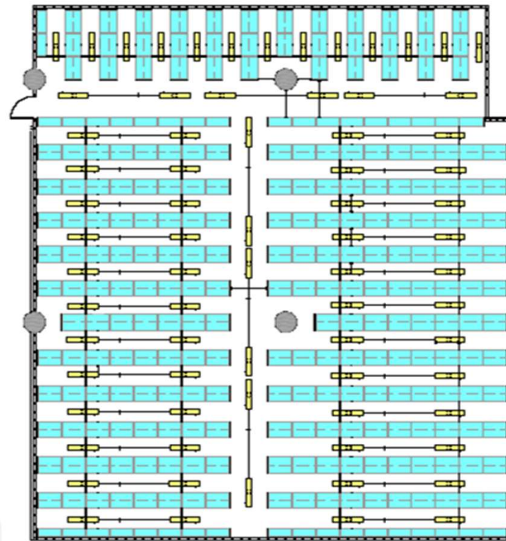
圖25 照明燈具安裝方向(固定式檔案架)
