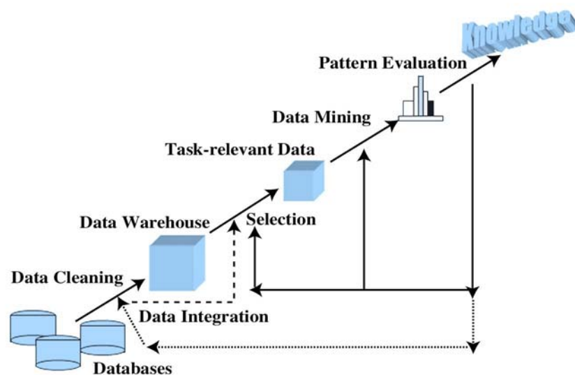
圖二 資料探勘的程序
