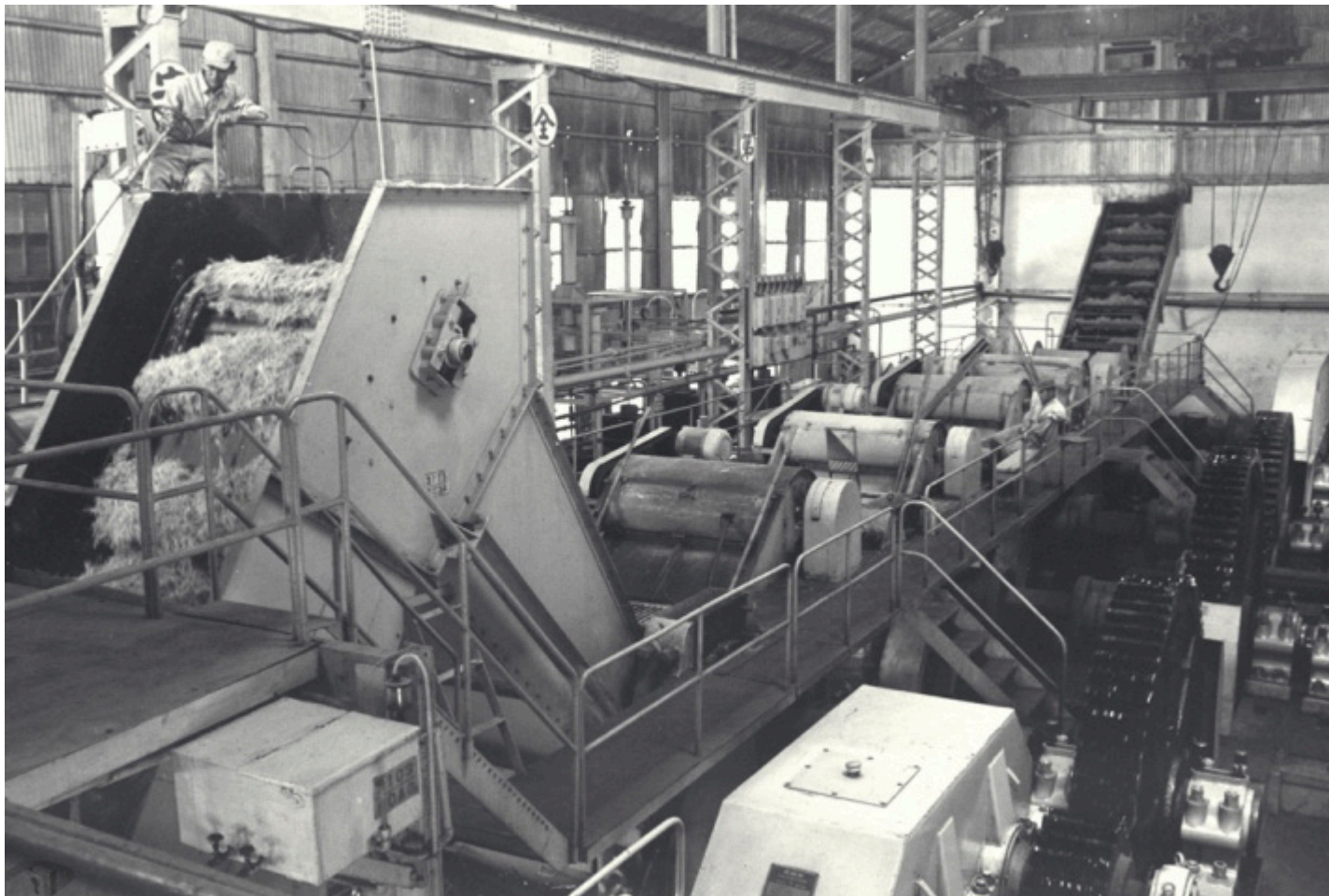
圖1 壓榨甘蔗汁的四重壓榨機
