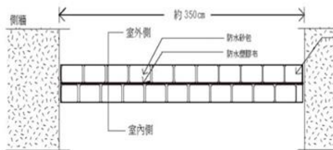
防水砂包堆置方式平面示意圖
