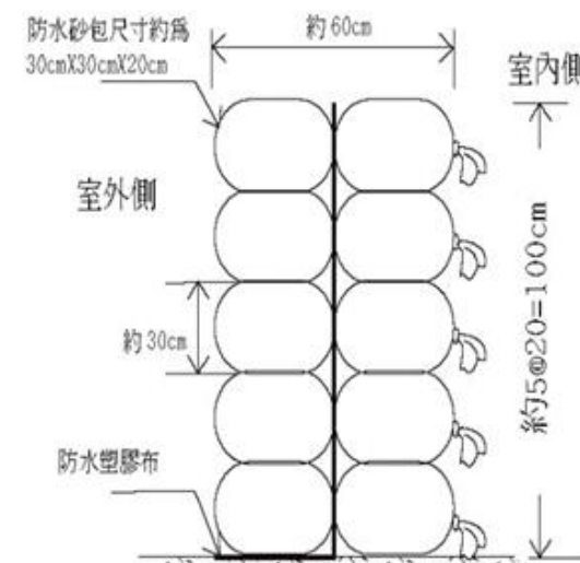
防水砂包堆置方式剖面示意圖
