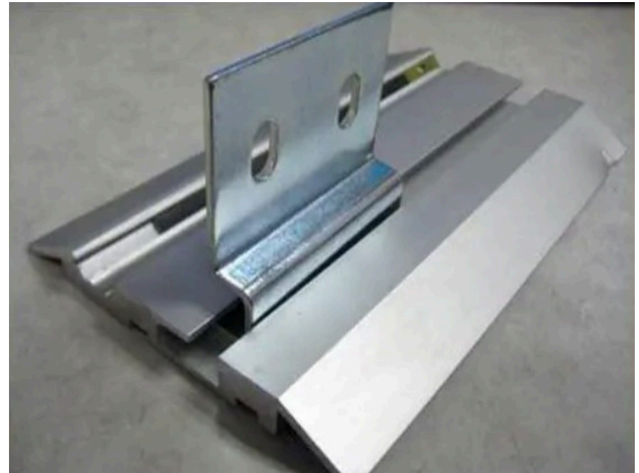
圖9 L型片狀卡榫
