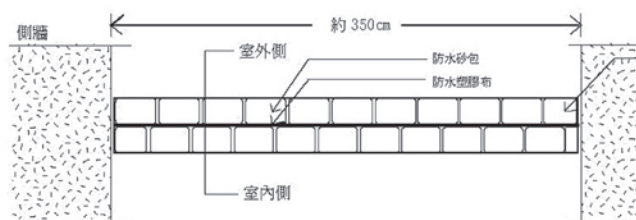
防水砂包堆置方式平面示意圖
