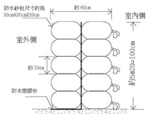
防水砂包堆置方式剖面示意圖
