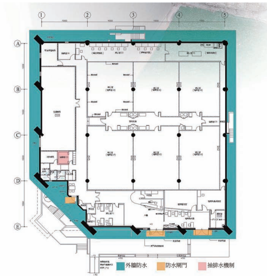
圖 57 防水機制示意圖
