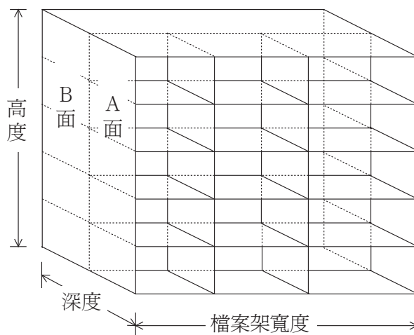
圖 76 檔案架高深寬示意圖
