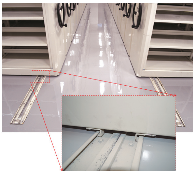
圖 80 密集式檔案架防傾倒卡樁示意圖
